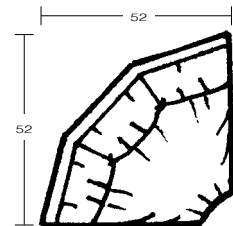
3549 WEDGE H36 W72 D39 INSIDE: H17 W50 D22 SEAT H: 20
